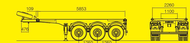
4 travas para 1 container 20'
