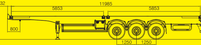
8 travas para 1 container 40' ou 2 containers 20'.
