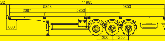
12 travas para 1 container 40' ou 2 containers 20' ou 1 container 20' centralizado.
