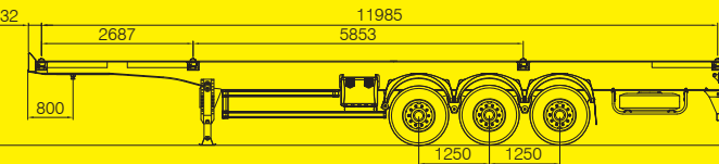
8 travas para 1 container 40' ou 1 container 20' centralizado.
